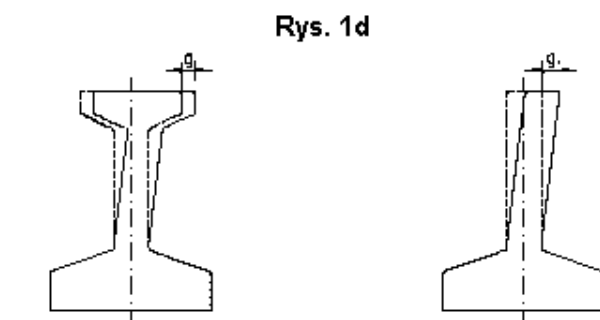
Rys. 1 - Główne wymiary i odchyłki
