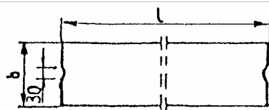
Rys. 1. Wymiarowanie Tablica 1. Wymiary krawężników betonowych
